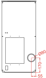
Vista da dietro - Rear view - Vue de derrière
