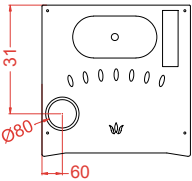
Vista da sopra - Top view - Vue de dessus
