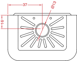
Vista da sopra - Top view - Vue de dessus
