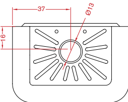
Vista da sopra - Top view - Vue de dessus
